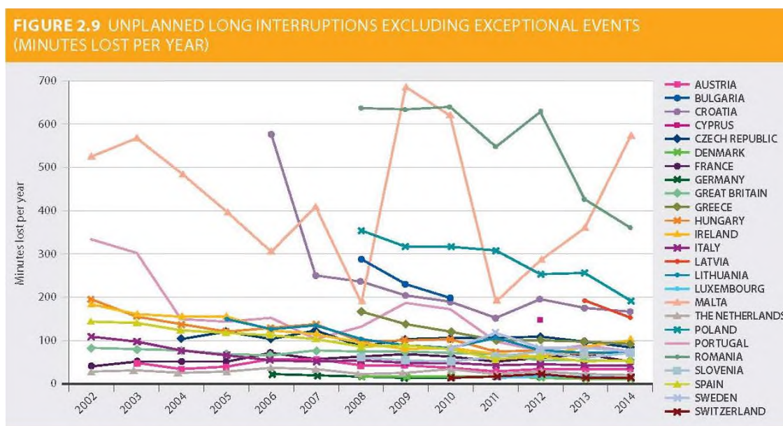
Figura 15. Valorile indicatorului SAIDI în țările UE (calculate cu excluderea întreruperilor cauzate de evenimente excepționale)
