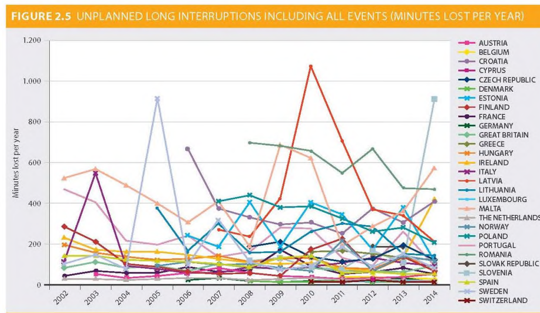
Figura 14. Valorile indicatorului SAIDI în țările UE (calculate pentru toate întreruperile neprogramate)
