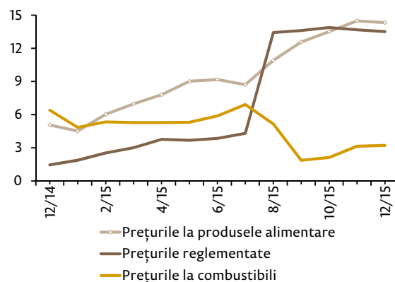
Graficul 2.22: Rata anuală a subcomponentelor inflației (%)
