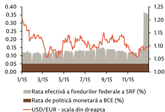
Graficul 1.2: Evoluția zilnică a USD/EUR
