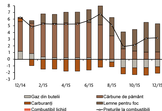
Graficul 2.27: Contribuția componentelor (p.p.) la creșterea anuală a prețurilor la combustibili (%)
