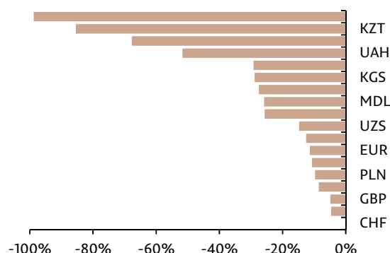
Graficul 3.32: Evoluția monedelor unor parteneri comerciali principali ai RM și a unor țări din regiune față de dolarul SUA (finele 2015), 31.12.2014 = 100
